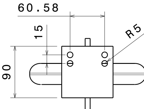
Top view Scale: 1:4
